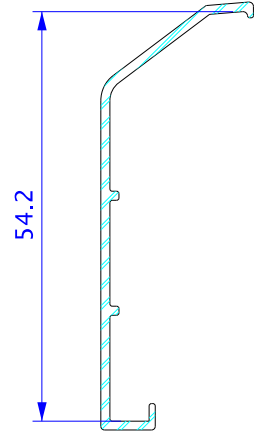
11534 =>10102 Dış
