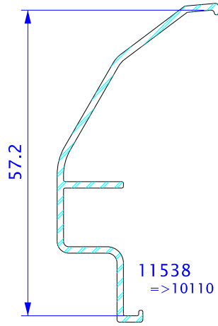
11537 =>10110 Düz
